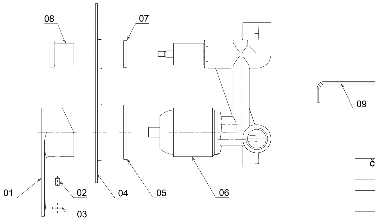
Rozložený stav
