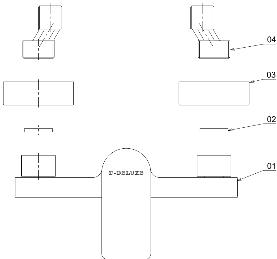
Rozložený stav
