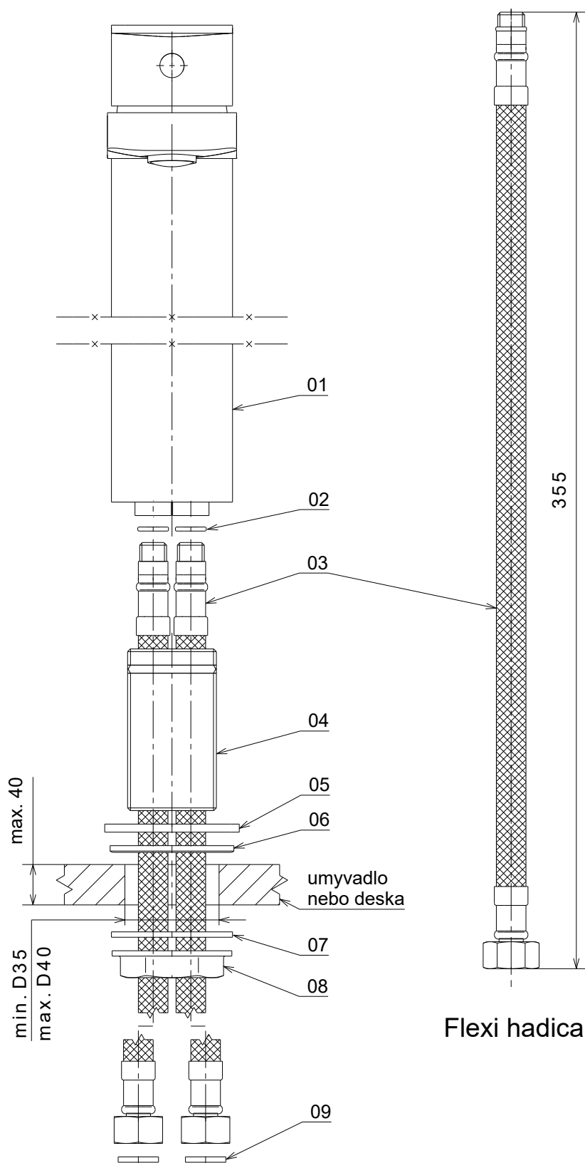
Rozložený stav
