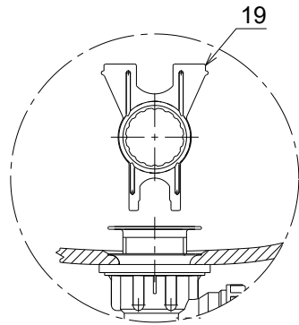
Použitie univerzálneho montážneho kľúča
