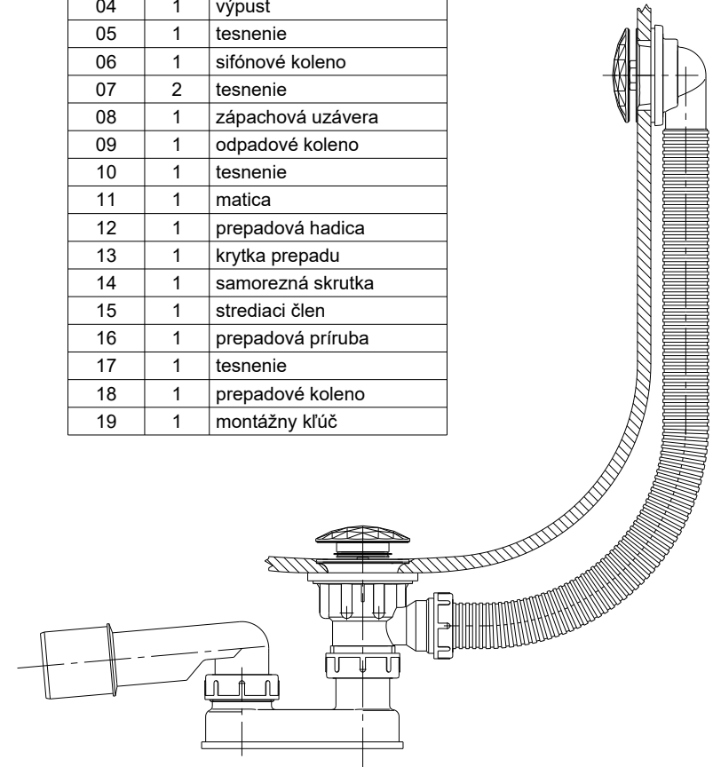
Zmontovaný stav
