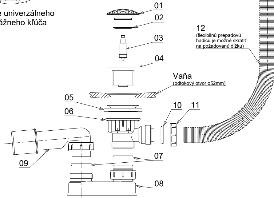
Rozložený stav
