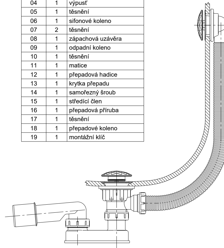
Smontovaný stav
