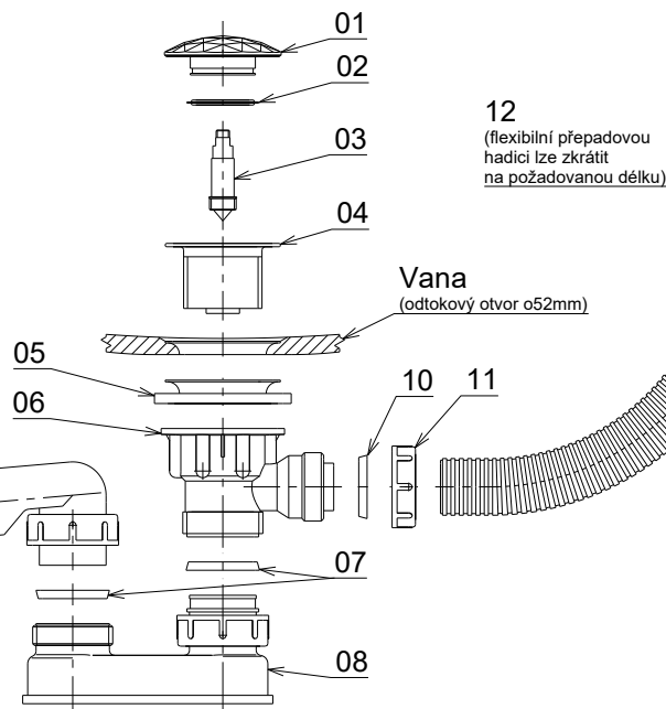
Rozložený stav
