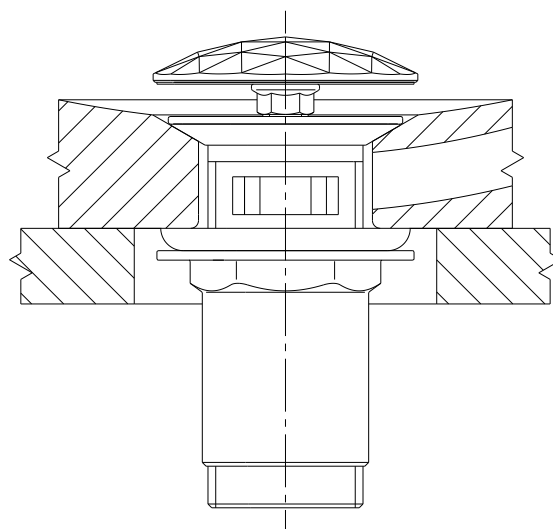
Zmontovaný stav
