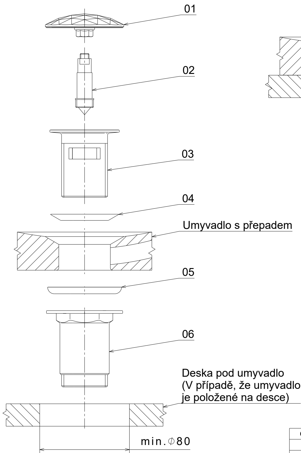
Rozložený stav
