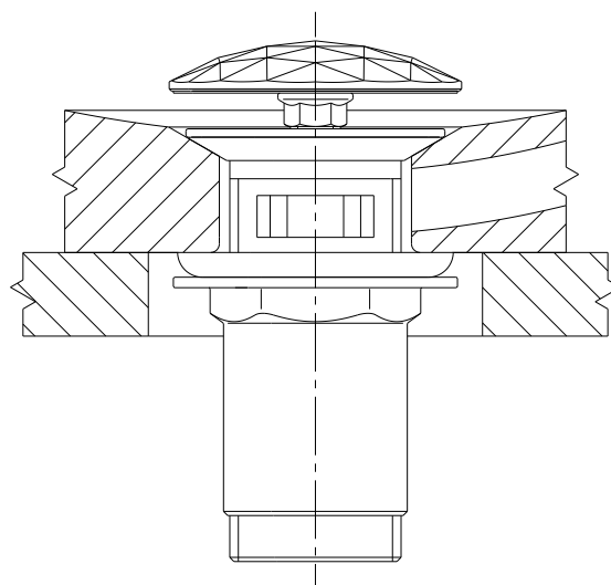
Smontovaný stav
