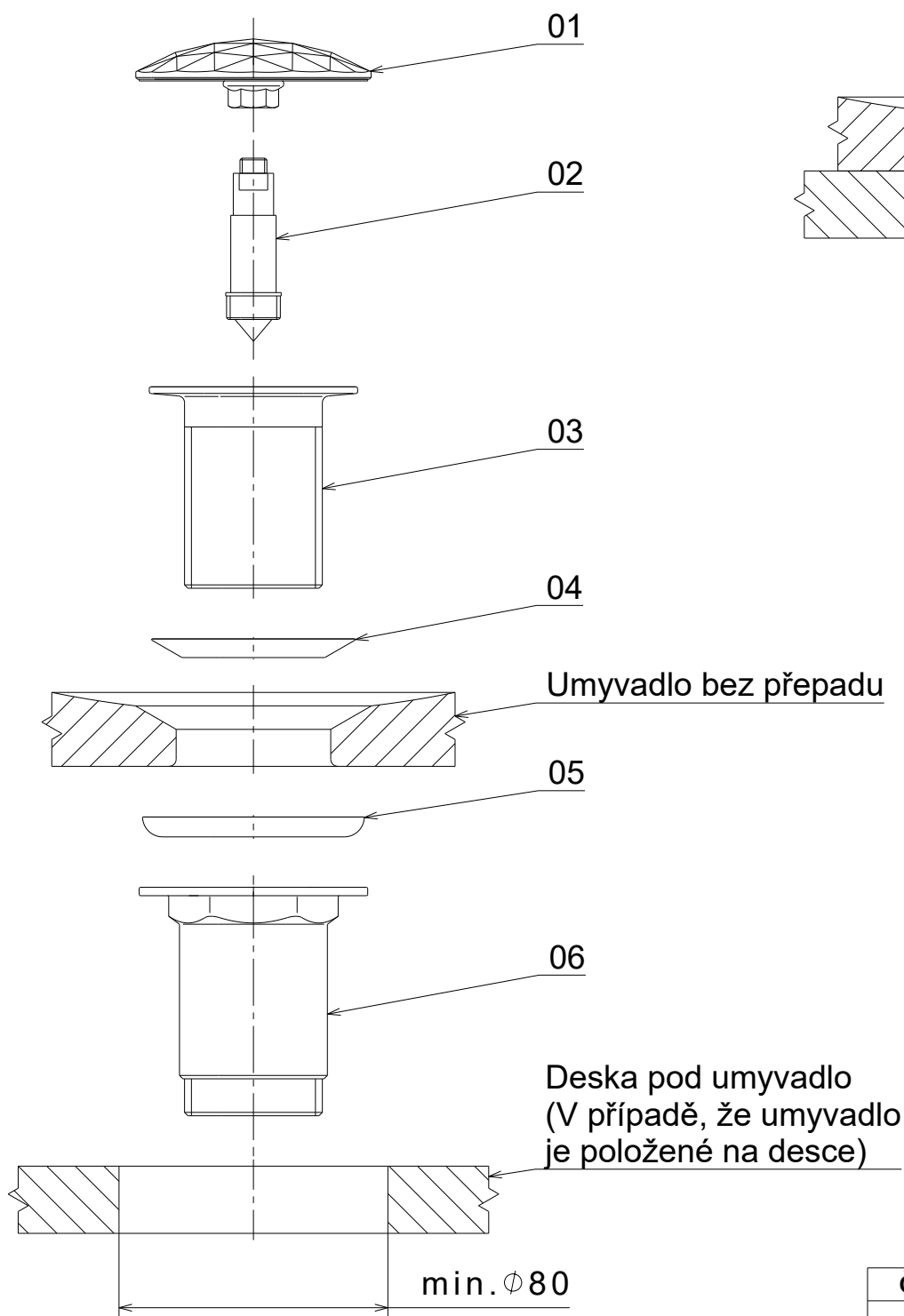
Rozložený stav
