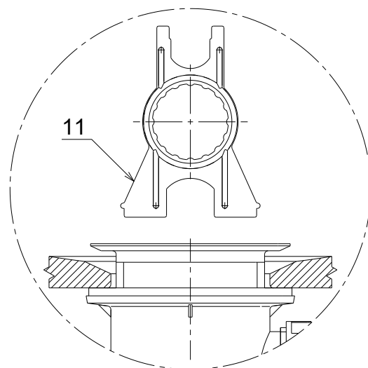
Použitie univerzálneho montážneho kľúča
