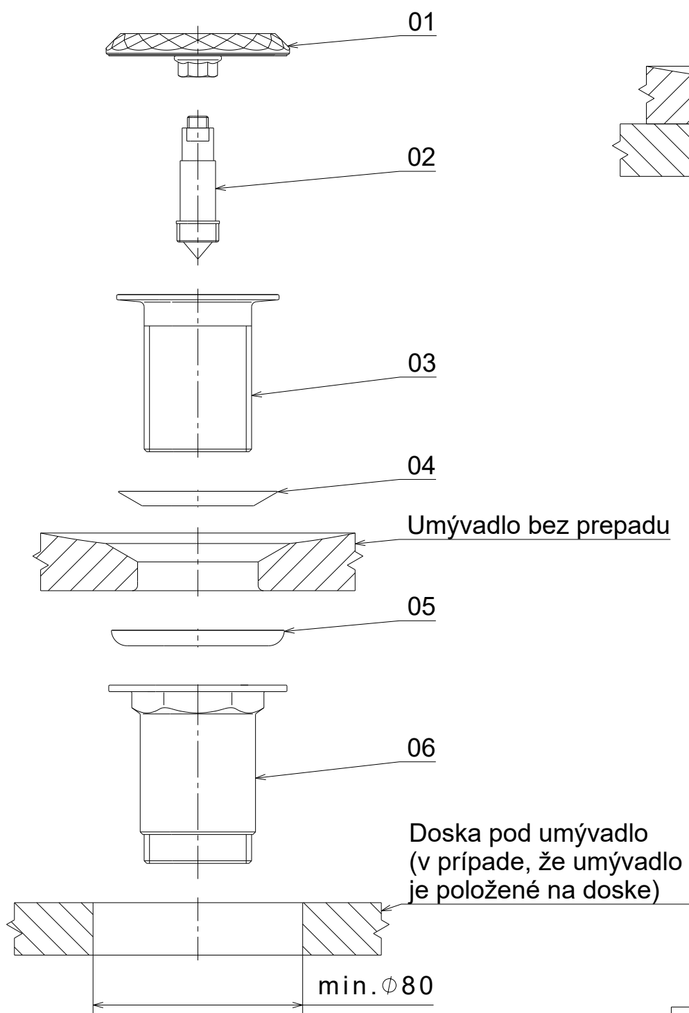
Rozložený stav
